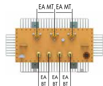
Encombrement Transformateur NOVARE Résidentiel avec bornes embrochables normales
